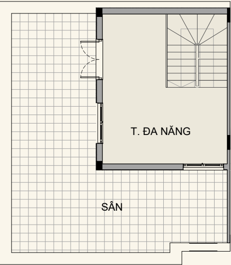
MẶT BẰNG TẦNG 4
