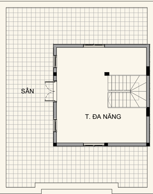
MẶT BẰNG TẦNG 2
